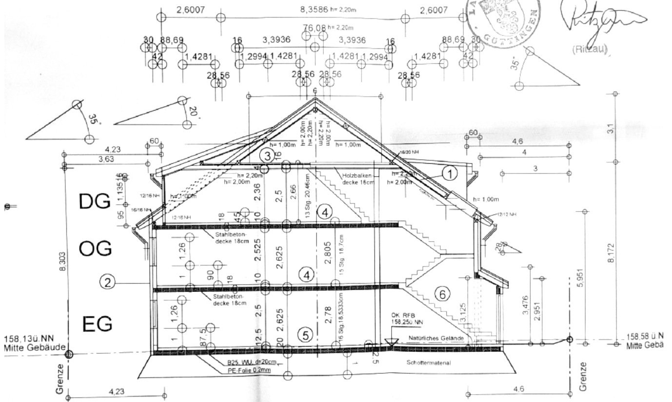
Querschnitt A-A
